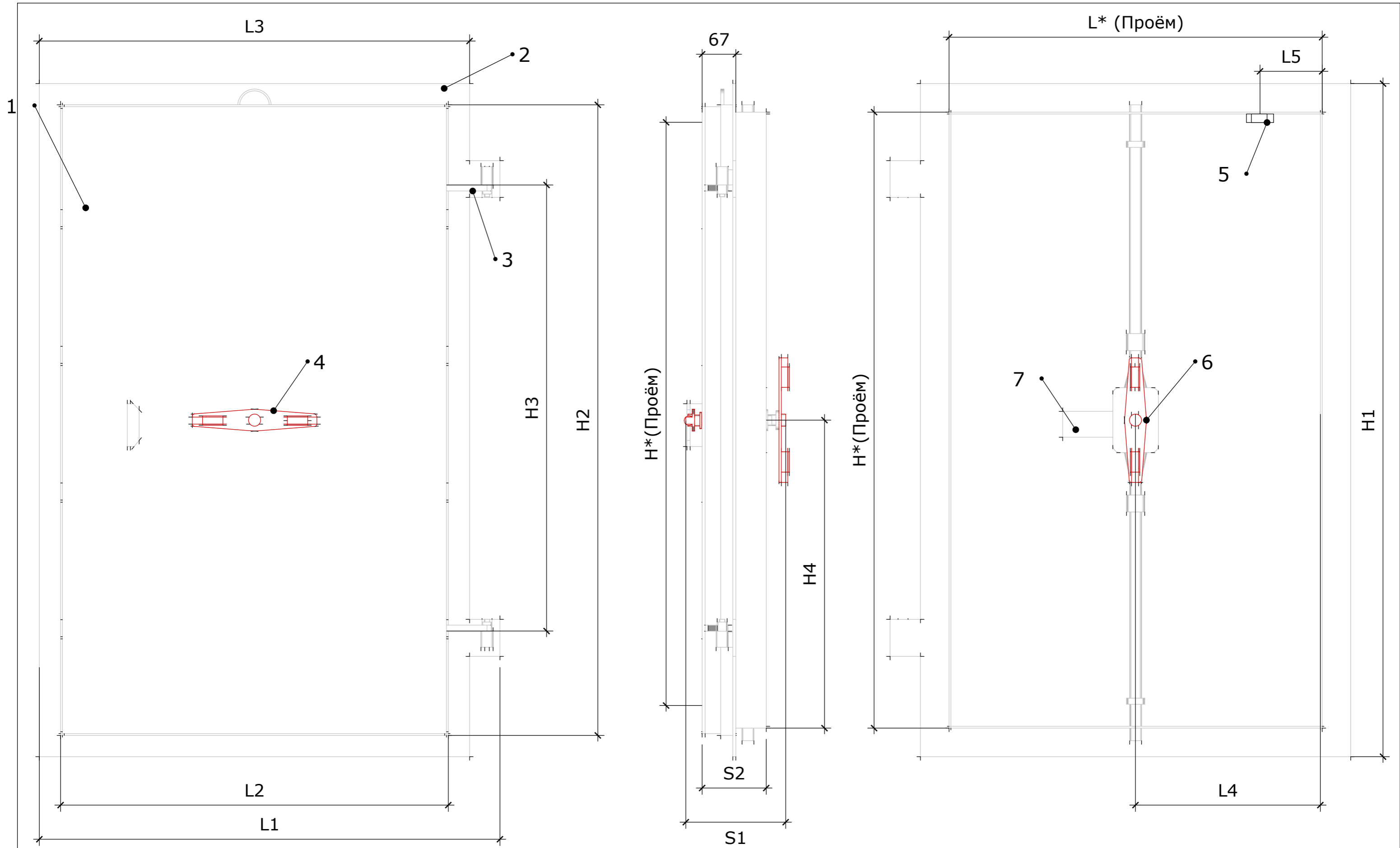
1. Полотно в сборе, 2. Коробка, 3. Петля в сборе, 4. Штурвал, 5. Сигнализации, 6. Механизм заdraивание, 7. Блокировочное устройство
